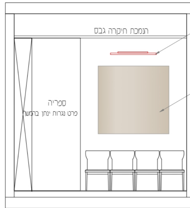
פריסה 10 קיר עזרת השנים
